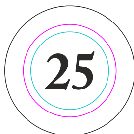
viditelná plocha 21mm grafika 25mm výsek 31mm
